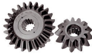
Crown Pinion H/D 13x23 Part No. NR 4302
